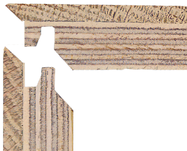
INNESTO A DOPPIO DENTE PER UNA PERFETTA TENUTA ANCHE SU GRADINI LARGHI
